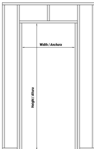
Height - Single Compact system inwards opening Altura - Sistema Compact Único con Apertura Interior
