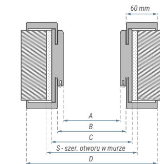
▼ Wymiary ościeżnicy do drzwi Natura HB PN23.
