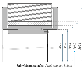
Falnyílás magassága / wall opening height
