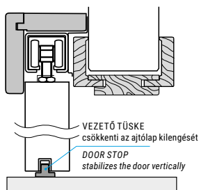
TOLÓAJTÓRENDSZER FÜGGŐLEGES METSZETI RAJZ
