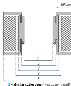
S - falnyílás szélessége / wall opening width
