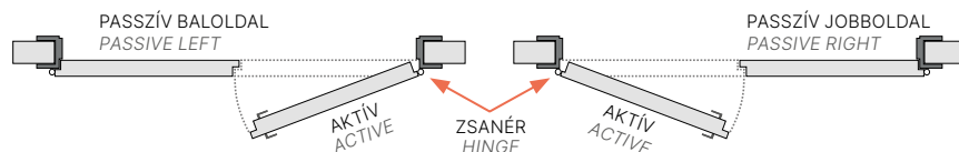
KÉTSZÁRNYÚ AJTÓ, JOBBS DOUBLE LEAF DOOR, RIGHT
