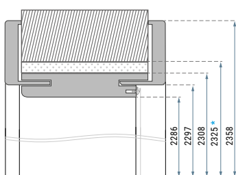
Ajtók méretek PN23 ajtóhoz. Dimensions of door frame for PN23 door.
