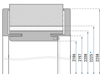
Ajtók méretei a PN22 ajtóhoz. Dimensions of door frame for PN22 door.
