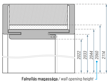
Falnyílás magassága / wall opening height
