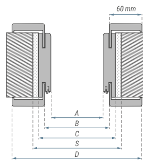
S - falnyílás szélessége / wall opening width
