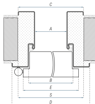
Wymiary ościeżnicy stalowej stałej PPOŻ [mm]
