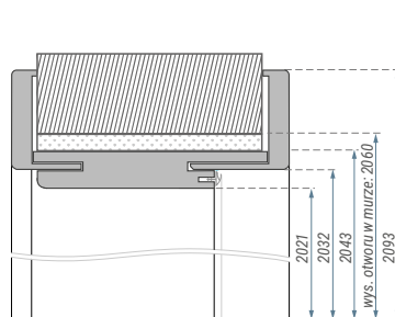
▼ Wymiary ościeżnicy do drzwi Natura HB PN22.
