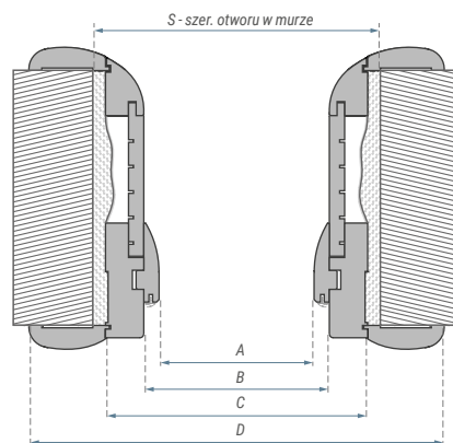
Wymiary ościeżnicy New Arcus [mm]:
