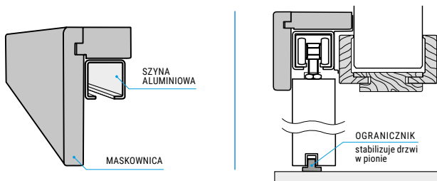
PRZEKRÓJ PIONOWY SYSTEMU PRZESUWNEGO
