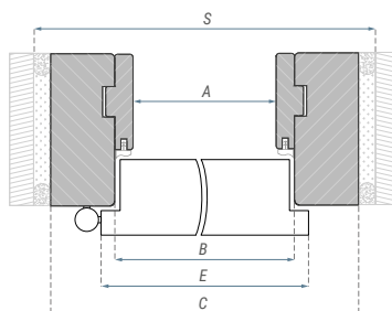
Wymiary ościeżnicy drewnianej stałej i regulowanej PPOŻ [mm]
