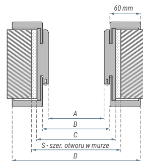
▼ Wymiary ościeżnicy do drzwi Natura HB PN23.
