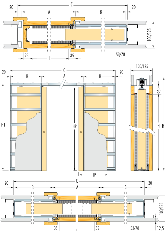
Tabulka rozměrů pro dvoukřídlové provedení Tabuľka rozmerov pre dvojkrídlové prevedenie
