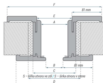
Rozměry reverzní zárubeň (mm) / Rozmery reverznej zárubne (mm)
