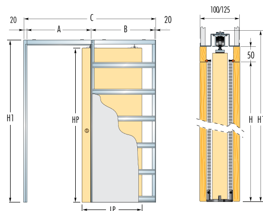
Tabulka rozměrů pro jednokřídlové provedení Tabuľka rozmerov pre jednokřídlové prevedenie
