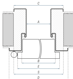
Wymiary ościeznicy stalowej stałej PPOŻ [mm]
