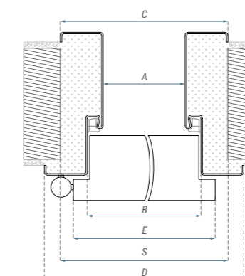
Размерите на BORD фиксирана каса на врата [мм]:
