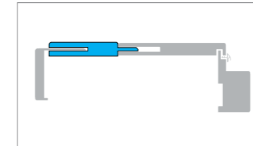
Вложка за регулиране 75 мм увеличава диапазон на регулиране: – в касата 70-110 мм до 150-185 мм – в касата 110-150 мм до 185-220 мм
