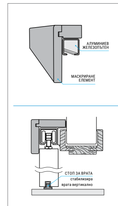
ВЕРТИКАЛНО СЕЧЕНИЕ НА СИСТЕМАТА ЗА ПЪЛЗАНЕ
