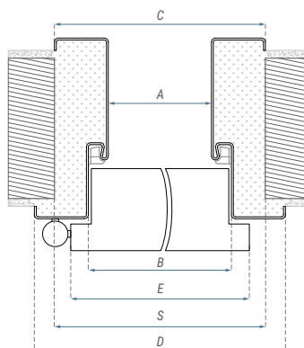
Wymiary ościeżnicy BORD stalowej stałej [mm]:
