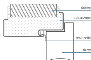
STAŁOWA STAŁA PRZYLGOWA ▼
