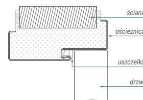
STAŁOWA STAŁA BEZPRZYLGOWA ▼
