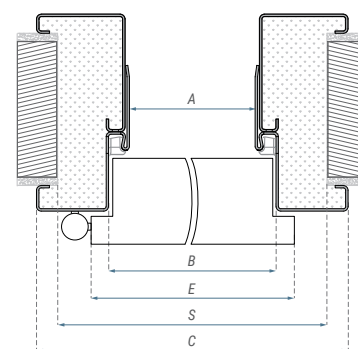
Wymiary ościeżnicy Regulowanej GUARD [mm]
