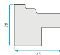
PROFIL LISTWY
