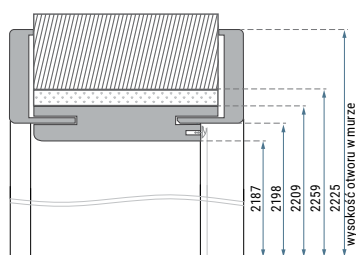
Wymiary ościeżnicy do drzwi PN22.
