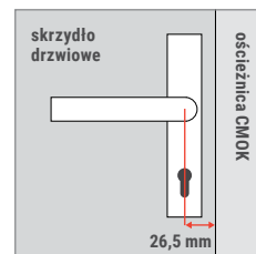
3. Wymiar klamki i rozety. Rączka klamki nie może wychodzić poza trzpień.
