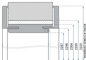
Wymiary ościeżnicy do drzwi PN23.
