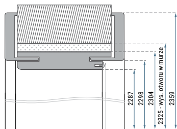
Wymiary ościeżnicy do drzwi PN23.
