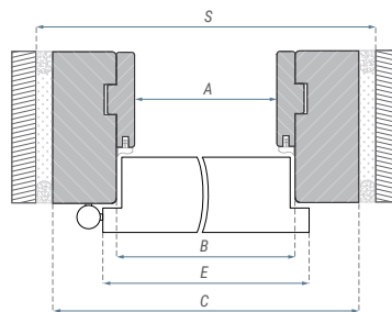
Wymiary ościeżnicy stałej PPOŻ [mm]
