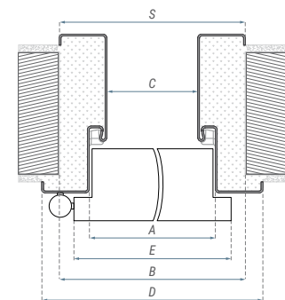
Wymiary ościeżnicy drewnianej PPOŻ [mm]
