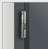
zawias czopowy drzwi przylgowych z regulacją 3D
