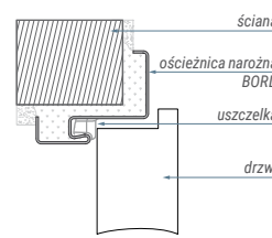
BORD STALOWA NAROŻNA STAŁA ▼
