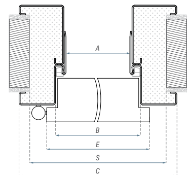
Wymiary ościeżnicy Regulowanej GUARD [mm]
