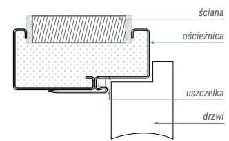
GUARD STALOWA REGULOWANA ▼
