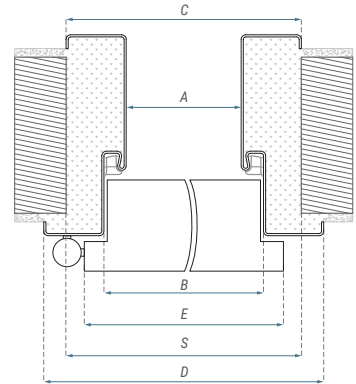
Wymiary ościeżnicy BORD stalowej stałej [mm]:
