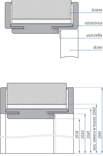
▲ OŚCIEŻNICA REGULOWANA BEZPRZYLGOWA
