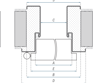
Wymiary ościeżnicy drewnianej PPOŻ [mm]
