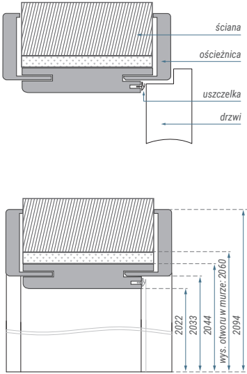
▲ OŚCIEŻNICA REGULOWANA
