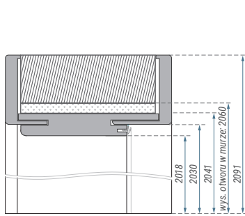
▼ OŚCIEŻNICA REGULOWANA BEZPRZYLGOWA 80
