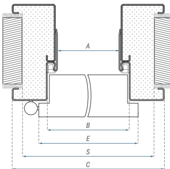
Wymiary ościeznicy Regulowanej GUARD [mm]
