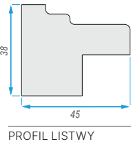
PROFIL LISTWY
