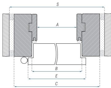
Wymiary ościeżnicy stałej PPOŻ [mm]
