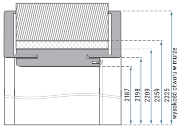
Wymiary ościeżnicy do drzwi PN22.
