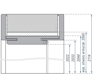
▼ OŚCIEŻNICA REGULOWANA 80
