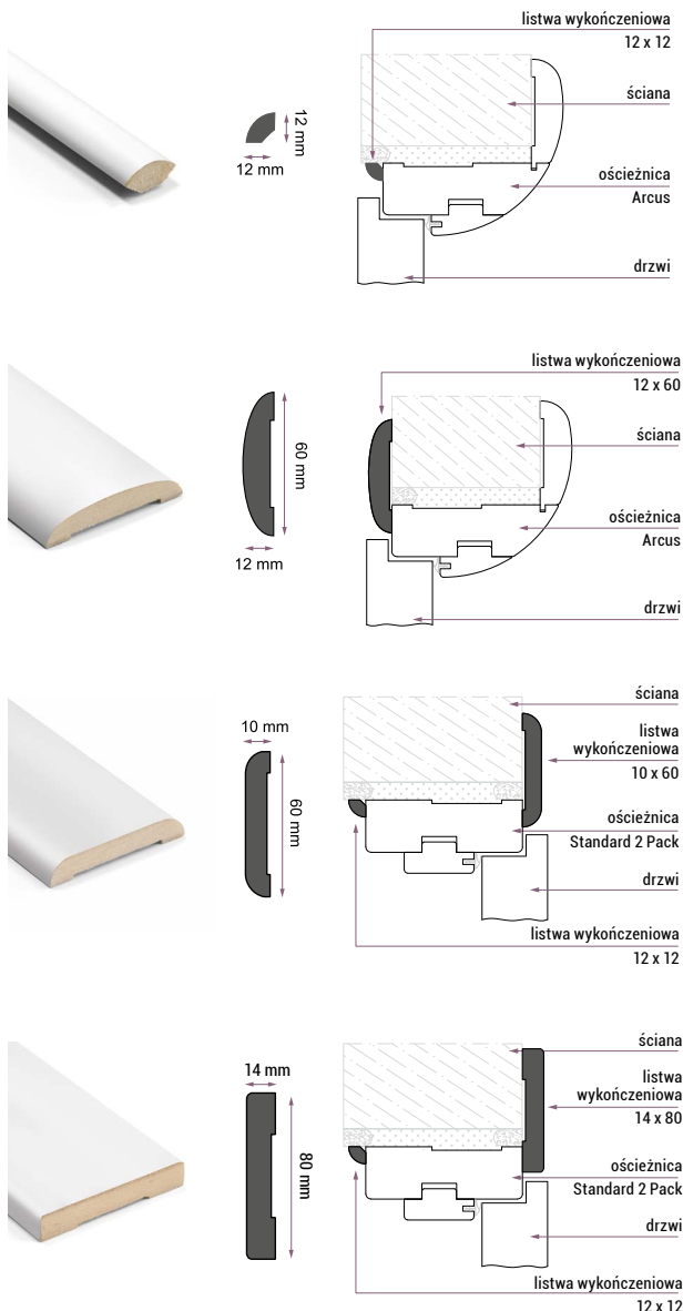
Listwa 14x80 mm jako listwa wykończeniowa oraz przypodłogowa.
