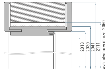
▼ OŚCIEŻNICA REGULOWANA BEZPRZYLGOWA 80
