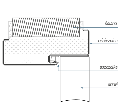
▲ OŚCIEŻNICA STAŁA STALOWA BEZPRZYLGOWA
