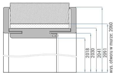
▲ OŚCIEŻNICA REGULOWANA BEZPRZYLGOWA
