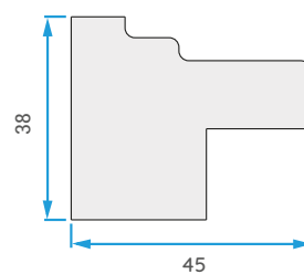
Profil listwy
