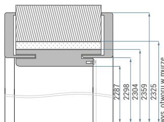
Wymiary ościeznica do drzwi PN23
