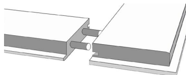
KONSTRUKCJA RAMOWA - elementy konstrukcji łączone za pomocą kołków montażowych
