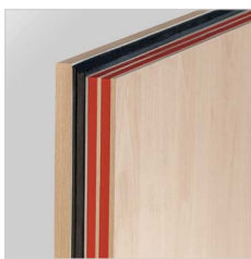
profil przyłgi DRZWI PRZYLGOWE
