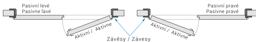
Dveře dvoukřídlé, pravé Dvere dvojkrídlé, pravé
