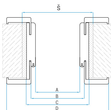
Rozměry obložkové zárubně bezfalcové (mm): Rozmery obložkovej zárubne bezfalcové (mm):
