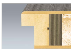
*) Konstrukce dveří profil Hard PF pro dekory CPL / Konštrukcia dverí profil Hard PF pre dekory CPL
