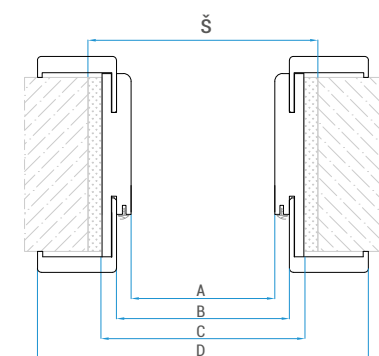
Rozměry obložkové zárubně bezfalcové (mm): Rozmery obložkovej zárubne bezfalcovej (mm):
