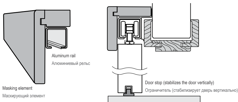
Vertical cross-section of the sliding system Вертикальное сечение раздвижной системы
