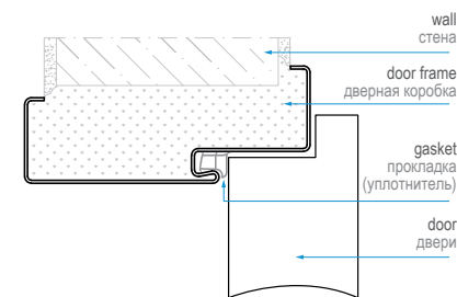
FIXED STEEL DOOR FRAME ФИКСИРОВАННАЯ СТАЛЬНАЯ
