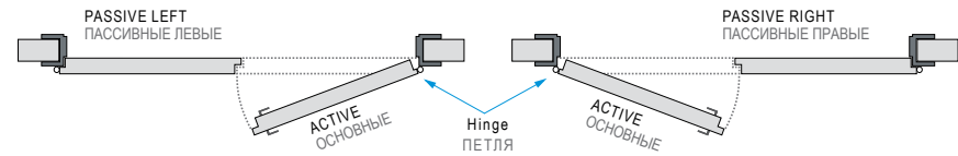
Double leaf door, right Двери двустворчатые, правые
