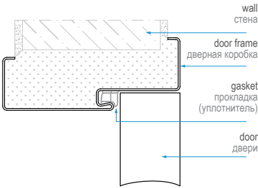
FIXED STEEL NON-REBATED DOOR FRAME ФИКСИРОВАННАЯ СТАЛЬНАЯ БЕЗ ПРИТВОРА
